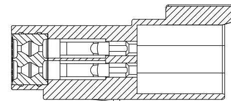
SEC A-A
