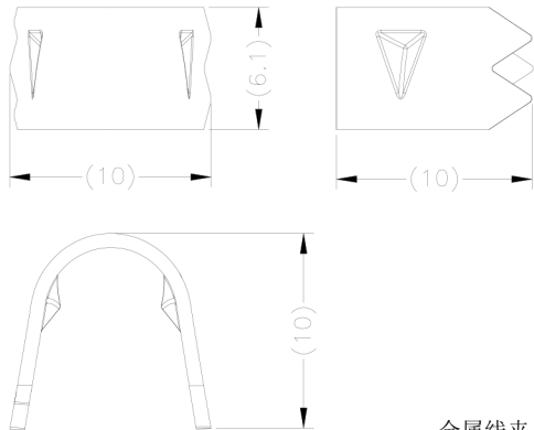
金属线夹:
